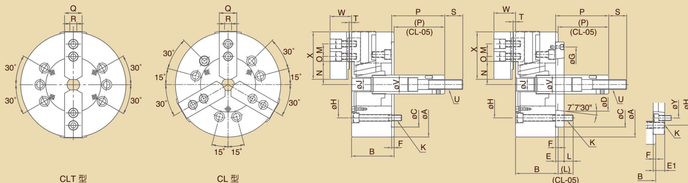
寸法図 >> Dimensions
